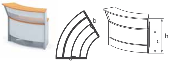
модуль наружный 60°
