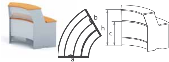
модуль внутренний 60°
