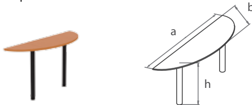
приставной элемент
